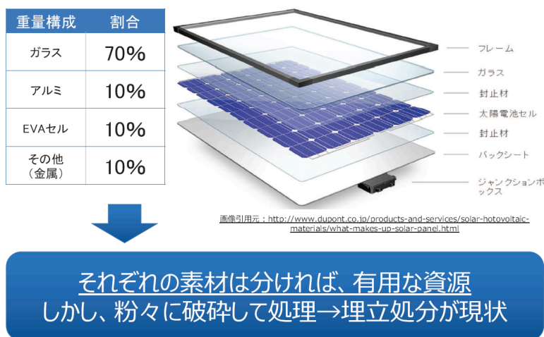
図8. 太陽光パネルの組成
