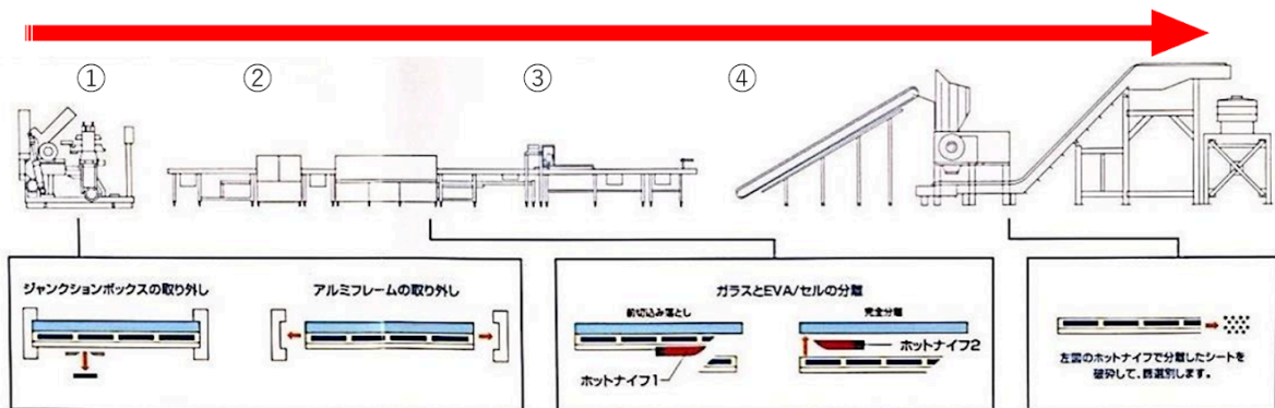
図12. 浜田のリサイクルフロー
