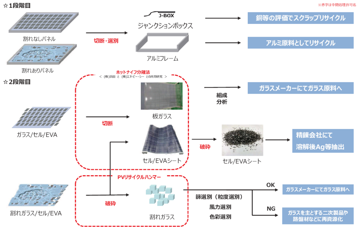
図11. 浜田のリサイクルフロー
